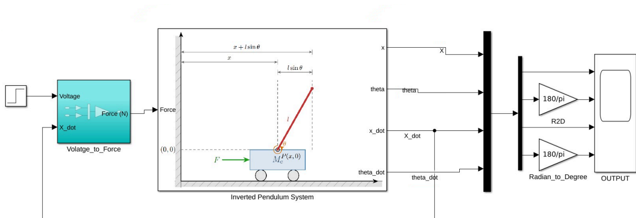
Figura 2: Model en llaç obert a Simulink.
