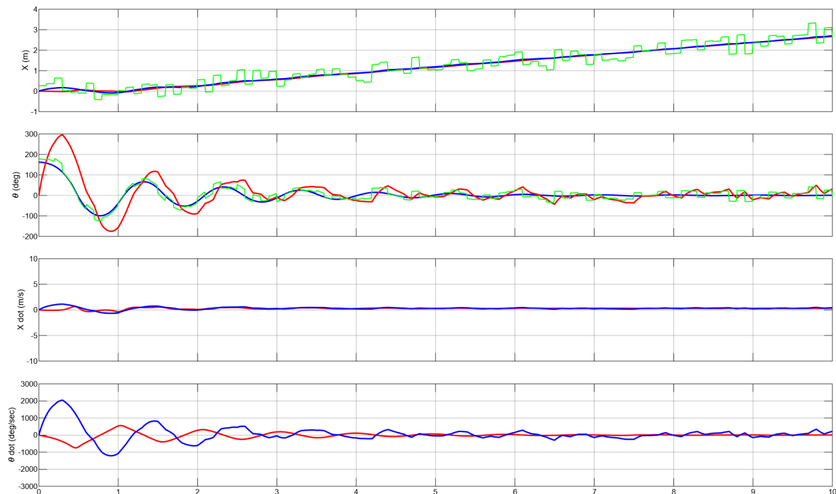
Figura 37: Cas 3 (sensors sorollosos). Estat real (vermell), estimació Kalman (blau) i mesura sorollosa (verd). Q_N/R_N = 0.01 .
