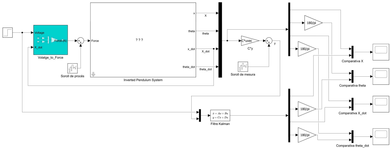
Figura 13: Diagrama Simulink de l'estimació d'estat amb el Filtre de Kalman. La planta no lineal rep com a entrada la força generada pel subsistema Voltage_to_Force . Només les sortides de posició i angle surten del bloc de la planta cap al Filtre de Kalman, al qual s'afegeix soroll de mesura. El bloc Kalman Filter reconstrueix els quatre estats estimats del sistema a partir d'aquestes dues mesures parcials.
